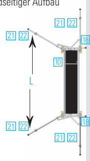
Wandseitiger Aufbau
